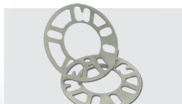
REF : 143 PAIRE CALES UNIVERSELLES • 3, 4 ou 5 trous de 98 à 120 d'entraxe • Dimensions : Épaisseur 3 mm
